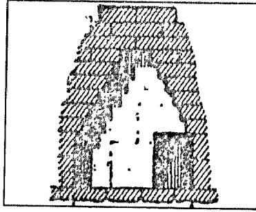
شكل (١٤) سقف مندرج (مصندوق Corbelling) من مصطنه من الاسره النايه عسره ندهسور .
